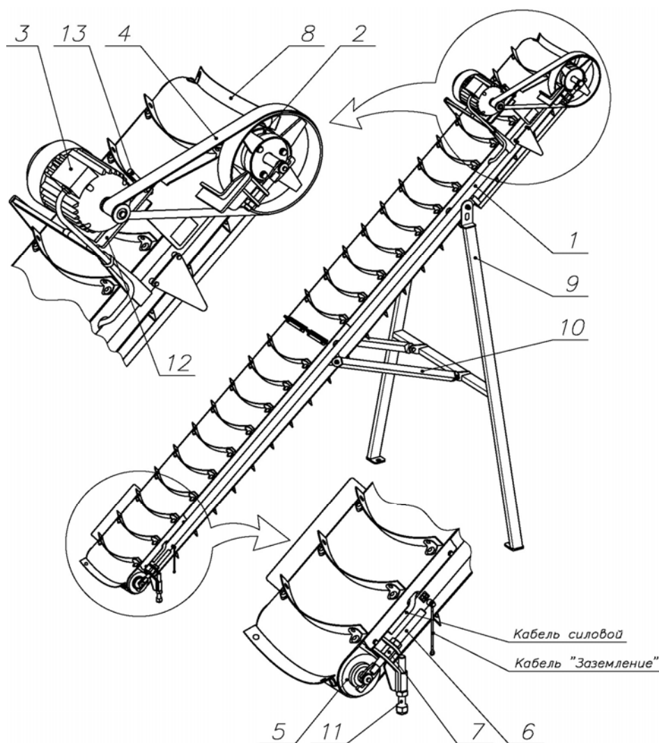
Рисунок 1. Транспортёр смеси.
