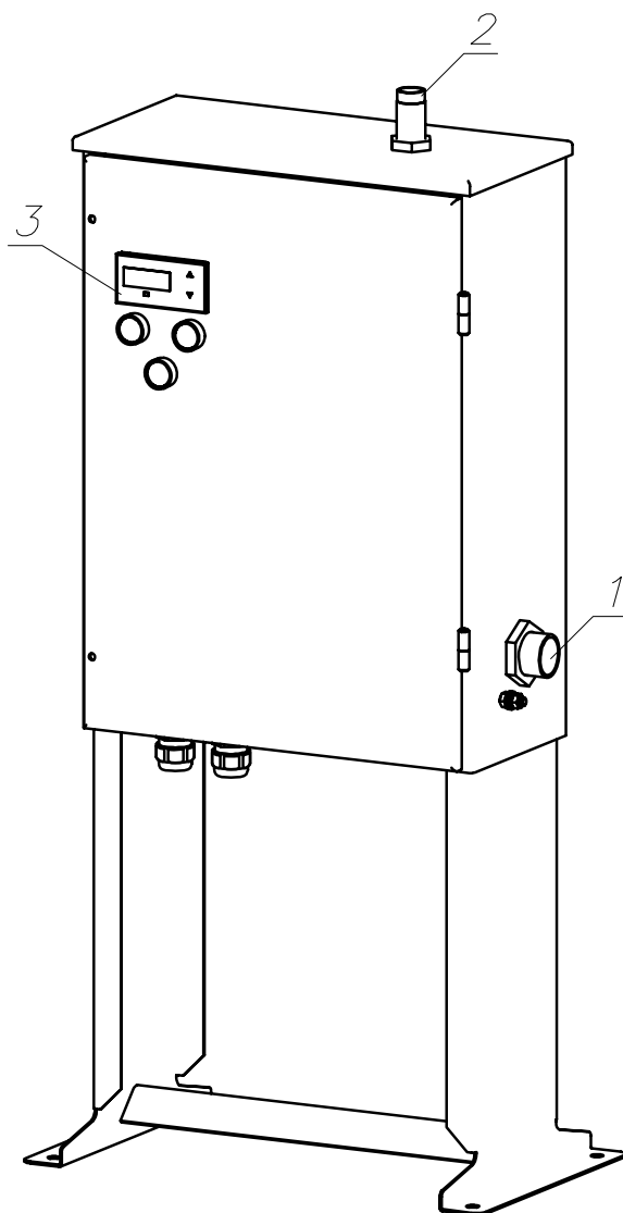
Рисунок 1 – Общий вид дозатора
