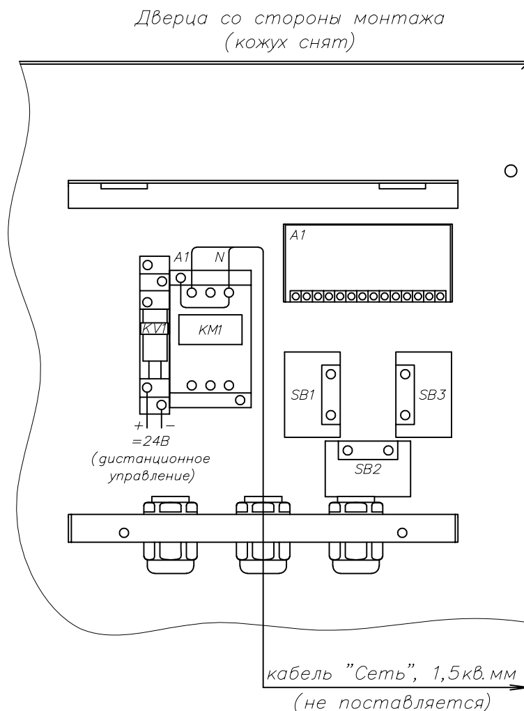
Рисунок 3 – Схема электрическая подключения
