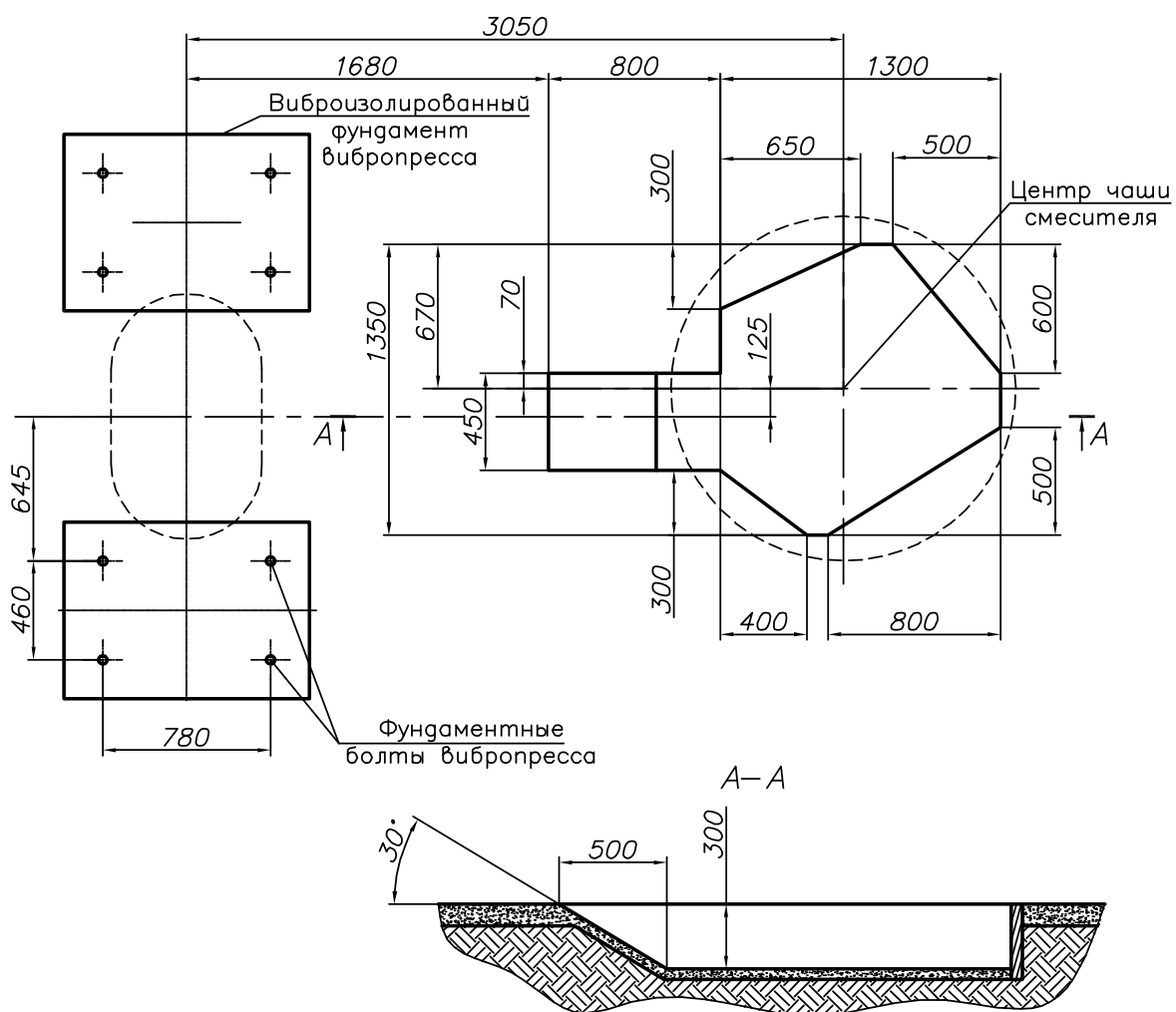
Рис. 17. Схема установки вибропрессов, бункера и смесителя в прямке.
