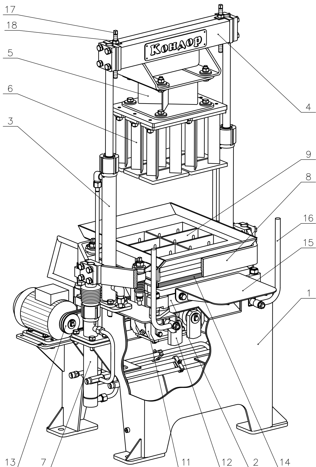
Рис.2. Вибропресс.
